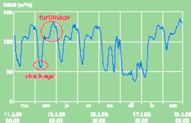
Fig. 1: Débit du Rhône à Branson (VS) au cours d'une semaine de février 2003 (11.2.-18.2.2003; Source OFEG). Encadrées de rouge et à titre d'exemple, les phases de stockage et de turbinage du 12.2.2003.
